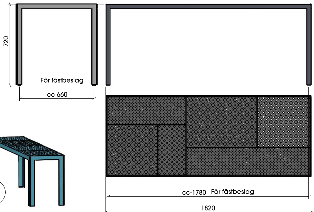
Montering av fästbeslag. Princip.
