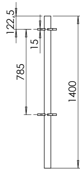
Vinkelstolpe 135°
