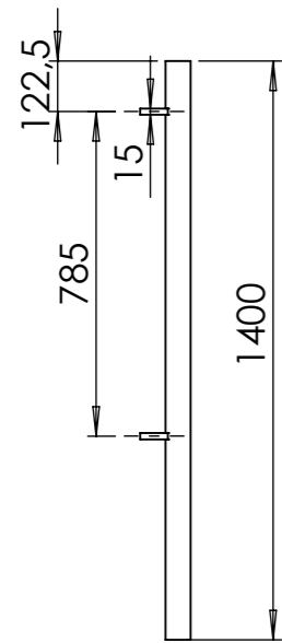
Slutstolpe
