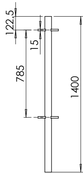
Mellanstolpe rak
