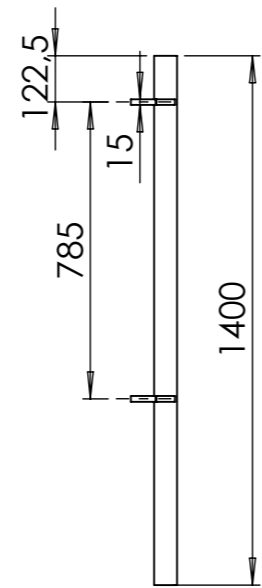
Vinkelstolpe 90°
