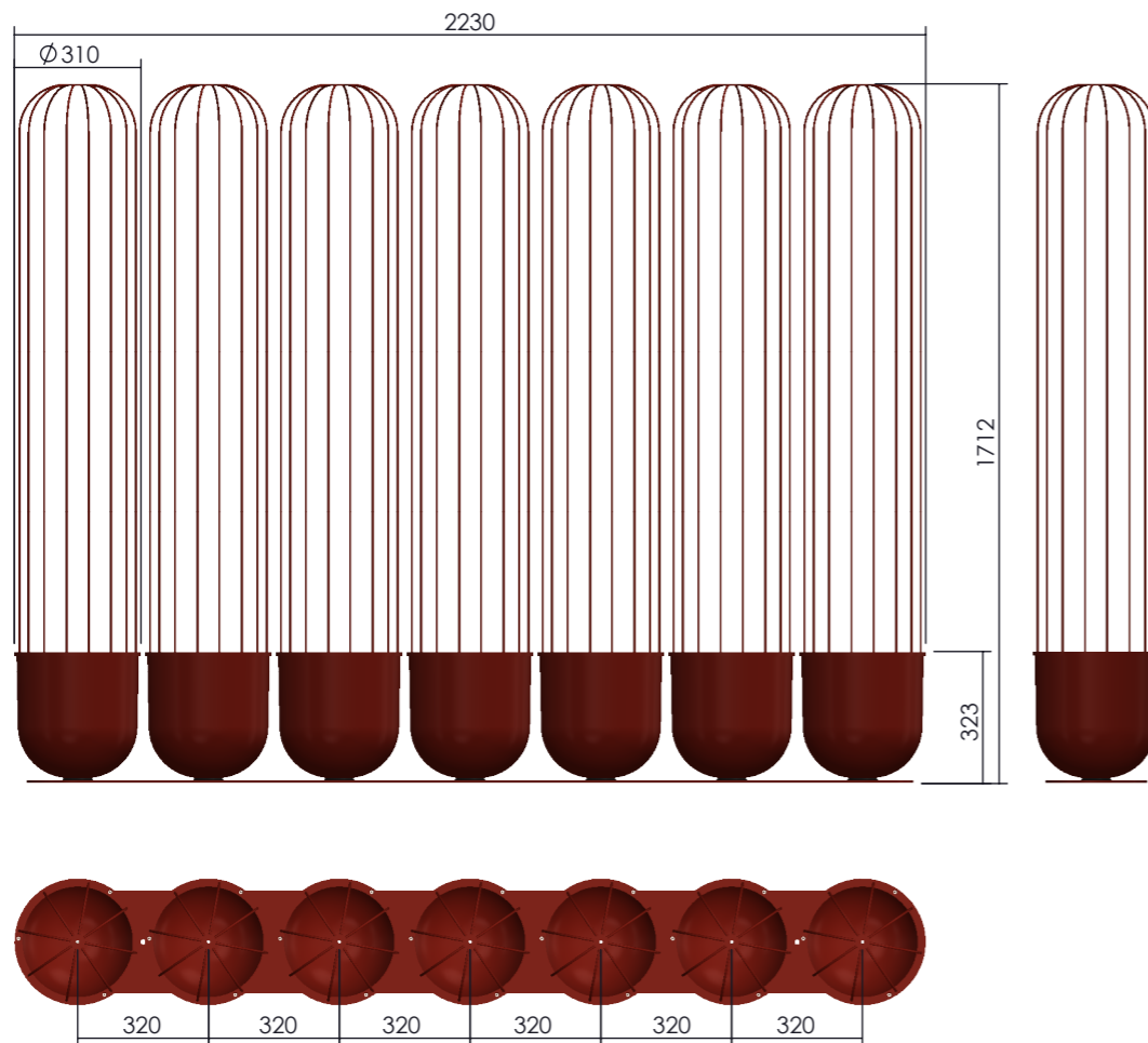
Grupp 3 Ö16-42/GR3 Vikt (oplanterad): 82 kg
