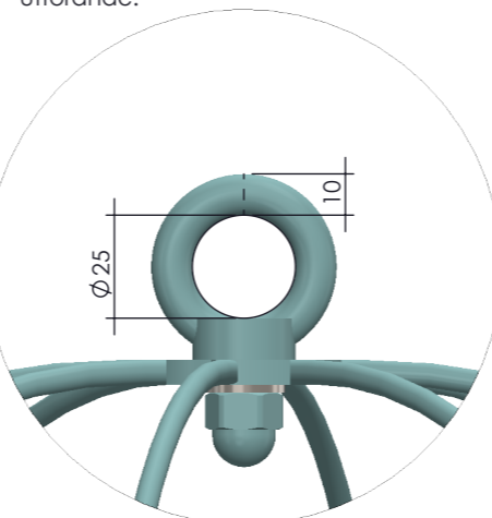
Detalj skala 1:2
