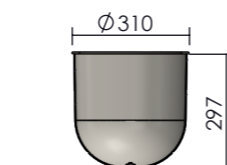
B-B Planteringskärl Ø 300 mm Effektiv öppning Ø270 mm Planteringsvolym ca 12 L
