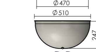
D-D Planteringskärl Ø 500 mm Effektiv öppning Ø470 mm Planteringsvolym ca 22 L
