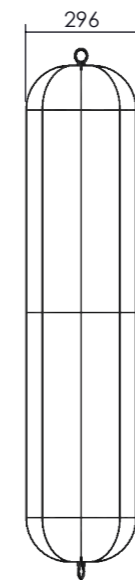
Kokong 1 Ö16-44/30 vikt: 3,5 kg
