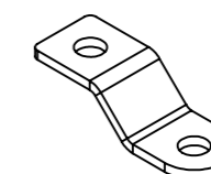
U80-81BESLAG Fastening bracket 1 pc
